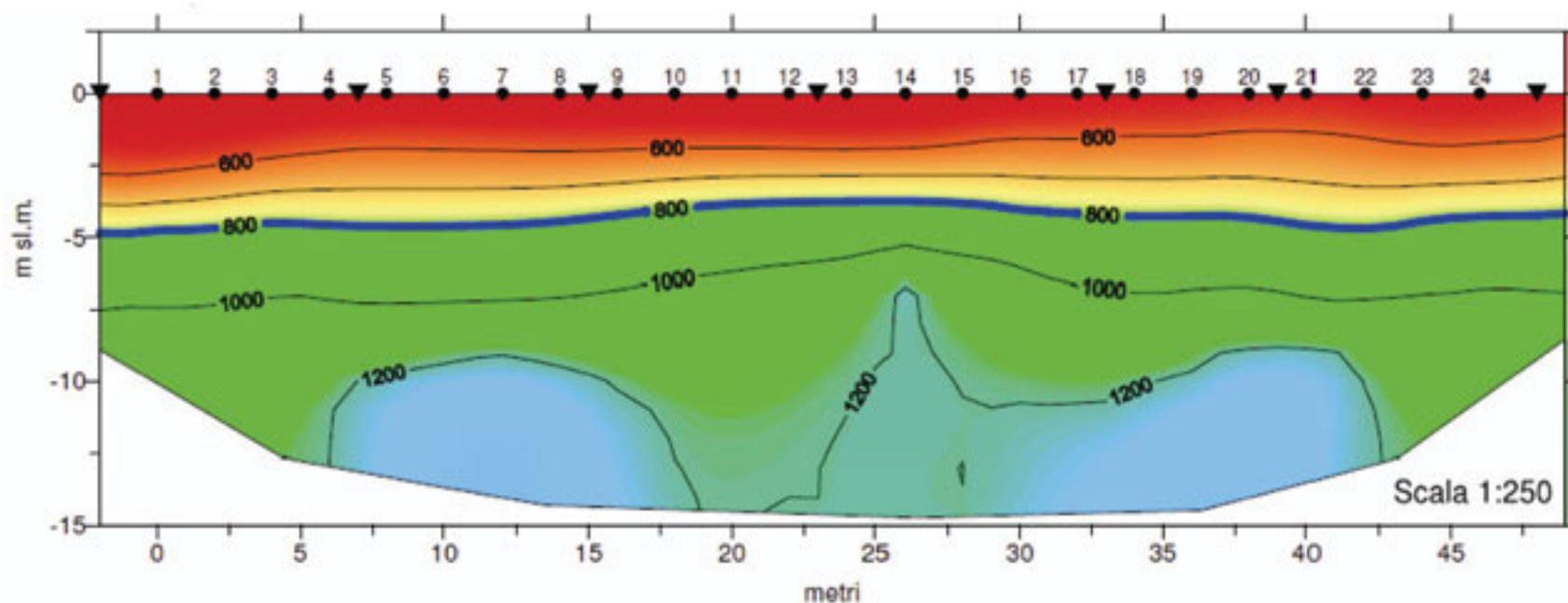
Fig. 1 – Esempio di sezione PRE-INIEZIONE ottenuta con tomografica sismica.
