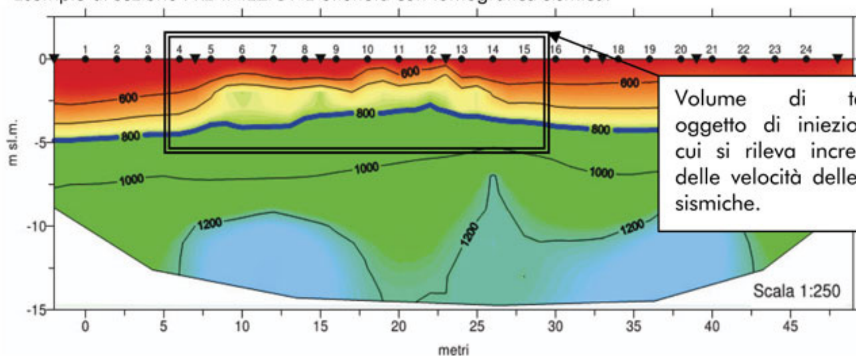
Fig. 2 – Esempio di sezione POST-INIEZIONE ottenuta con tomografica sismica, in cui la velocità delle onde sismiche rifratte è direttamente proporzionale alle caratteristiche geomeccaniche del substrato fondale.
